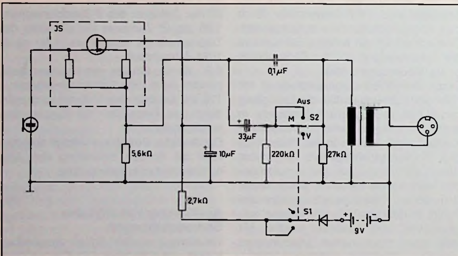
Bild 1: Schaltung des Electret-Mikrofon
