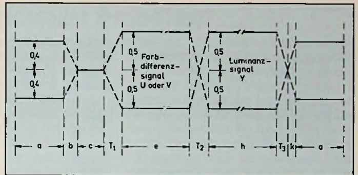
Bild 2: Kanalraster des D2-MAC-Farbfemsehsignales, Taktfrequenz = 20,25 MHz
