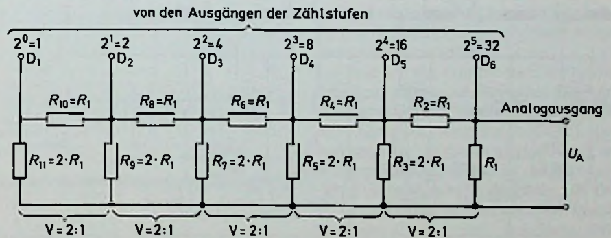
Bild 6.3: Kettenleiter-Netzwerk für D/A-Wandler
