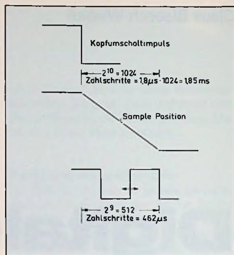
Bild 2: Ausgangssignale der Phasenvergleicherschaltung
