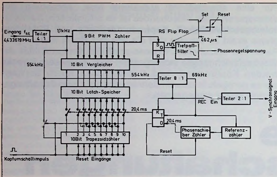
Bild 1: Prinzipschaltung der digitalen Kopftrommelphasenregelung
