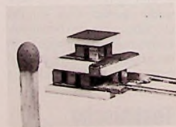
Bild 1: Peltier-Kühler zur elektronischen Kühlung von Halbleiterbauelementen (Nucletron-Pressbild)
