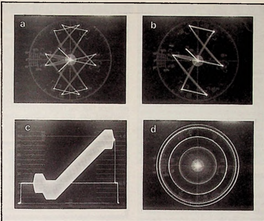
Bild 2: Vektor-Oszillogramme: a) komplette PAL-Darstellung, b) +V-Komponente wird dargestellt, geschaltete PAL-Komponente wird unterdrückt, c) Sägezahnsignal mit überlagertem Farbträger, d) Symmetriekontrolle mit freilaufendem Farbträger
