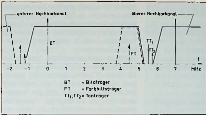
Bild 1: Kanalraster des PAL-Farbfemsehsignals BT = Bildträger, FT = Farbhilfsträger, TT1 = Tonträger 1, TT2 = Tonträger 2
